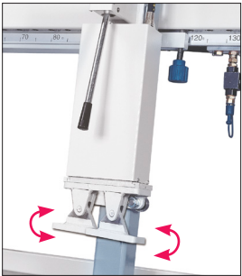
Otočné tlakové pätky pre naklonené rámy
