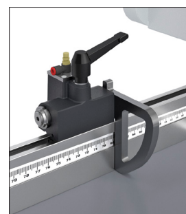
Pneumatický bočný doraz 60 mm (voliteľné).
